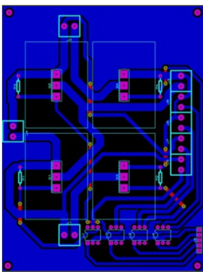
Figura 3. Placa del circuito de la etapa de potencia
