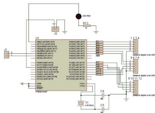
Figura 4. Diagrama eléctrico de la etapa de control.
