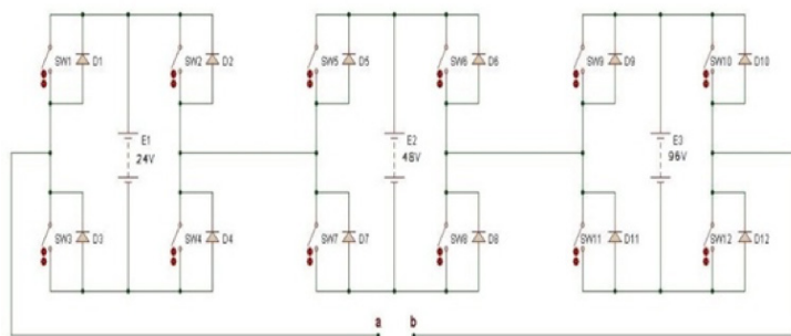
Figura 1. Esquema de conexiones
